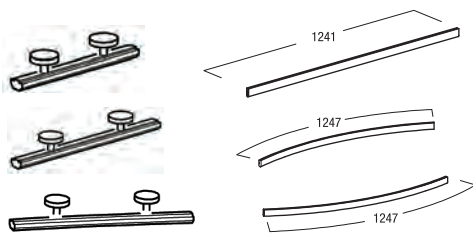
Zargen (M 1356) OP 181 Zarge gerade OP 183 Zarge konkav gebogen OP 185 Zarge konvex gebogen
